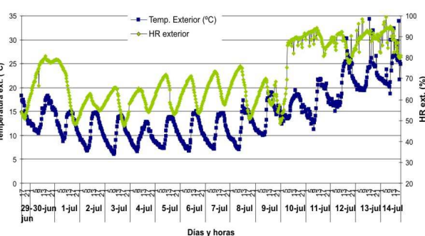
Figura 12b: Registros de temperatura exterior y HR ambiente en Resistencia, entre el 30/06/11 y el 14/07/11.
