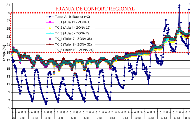
Figura 13: Evolución de temperaturas interiores en 6 aulas del edificio de la FAU - UNNE, durante el período del 30/06/2011 al 14/07/2011.
