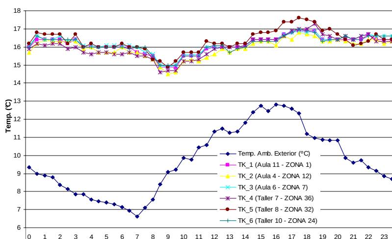
Figura 14: Evolución de temperatura interior en 6 aulas del edificio de la FAU, para el día 04/07/2011.
