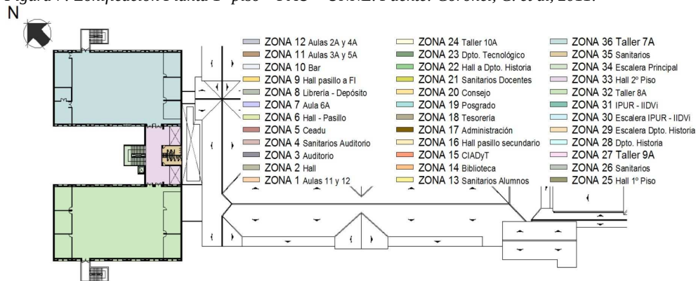
Figura 8: Zonificación Planta 2° piso – FAU – UNNE. Fuente: Coronel, C. et al, 2011.
