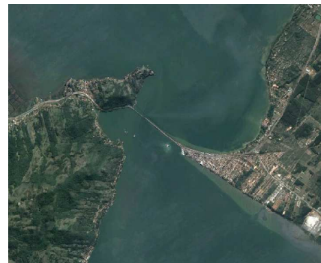
Figura 9. Vista de la maqueta computacional del Puente atirantado e identificación de la rugosidad del terreno por satélite.
