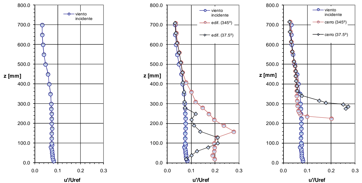
Figura 8. Perfiles de intensidad de turbulencia del viento incidente, en la posición del edificio y sobre los cerros.
