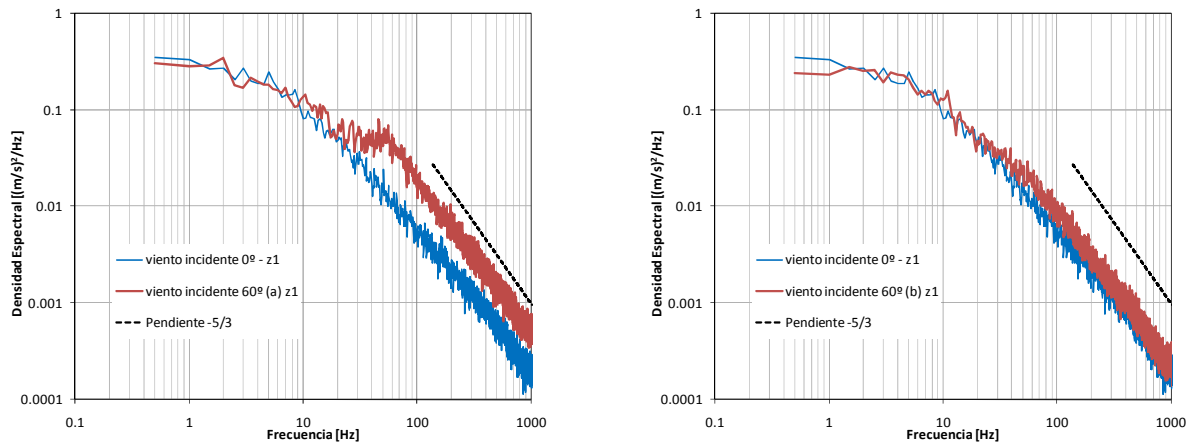
Figura 14. Comparación de los espectros en la región del puente para viento incidente 0^\circ y 60^\circ (a), a la izquierda, y 60^\circ (b), a la derecha – altura z_1 .
