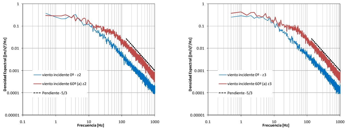
Figura 15. Comparación de los espectros en la región del puente para viento incidente en las direcciones de 0^\circ y 60^\circ (a) – alturas z_2 y z_3 .
