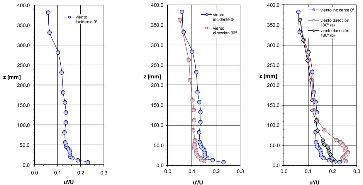
Figura 13. Perfiles de intensidad de turbulencia del viento incidente, en la dirección de 90^\circ y en la dirección de 180^\circ .
