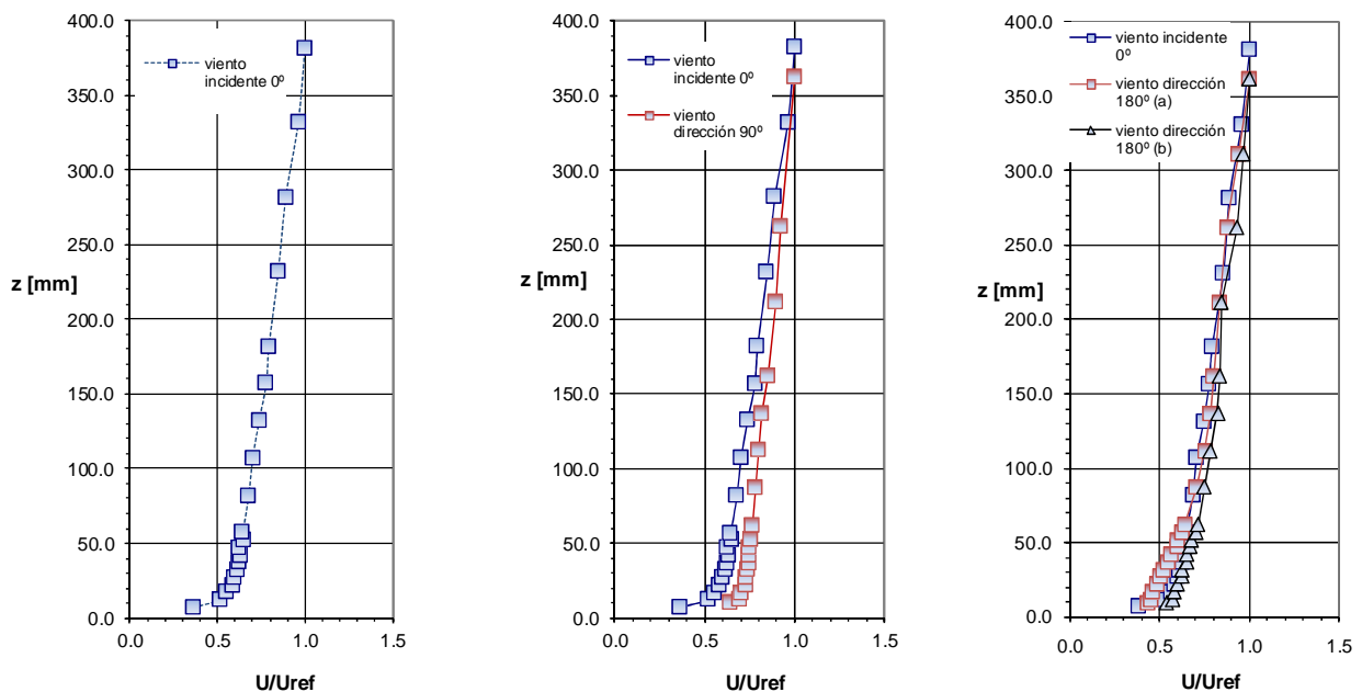
Figura 12. Perfiles de velocidad media del viento incidente, en la dirección de 90^\circ y en la dirección de 180^\circ .
