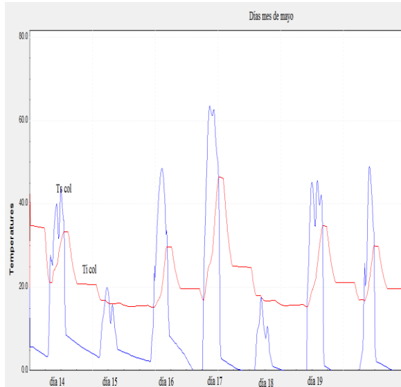
Figura 5: Variação da temperatura da água a la entrada y salida del colector
