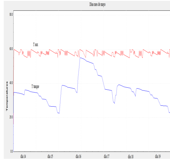
Figura 6: Variação da temperatura del agua en el tanque térmico y temperatura de la fuente auxiliar.
