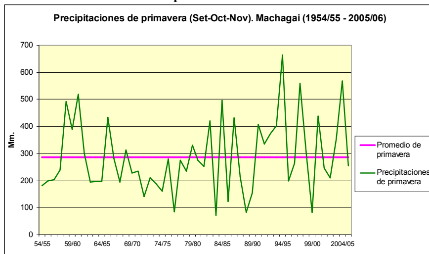
Gráfico N° 6: Precipitaciones en Primavera 1954-2006.
