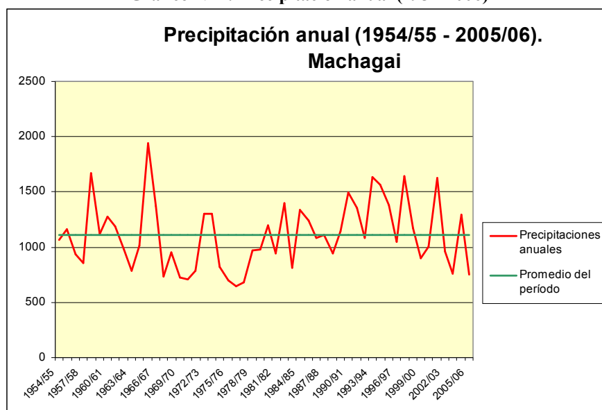
Gráfico N° 2: Precipitación anual (1954-2006)
