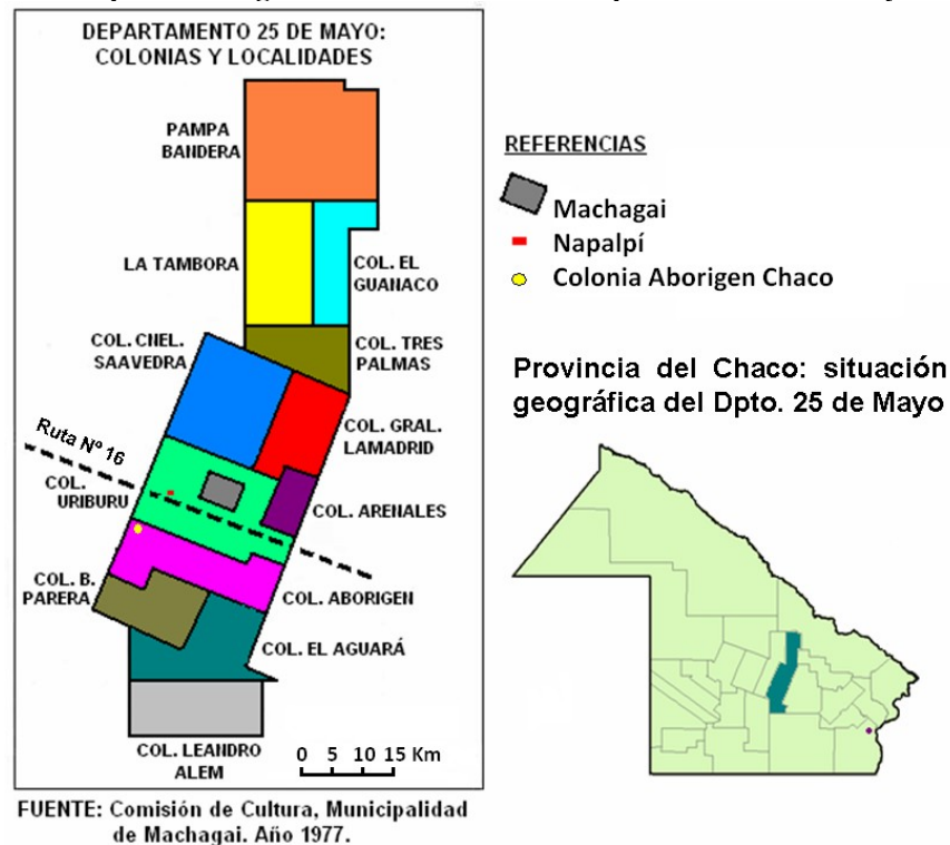
Mapa N° 2: Organización territorial del Departamento 25 de Mayo.
