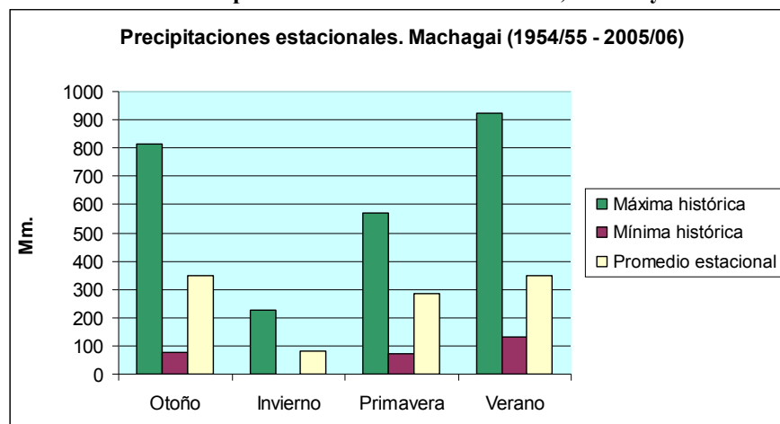
Gráfico N° 3: Precipitaciones estacionales máximas, medias y mínimas.
