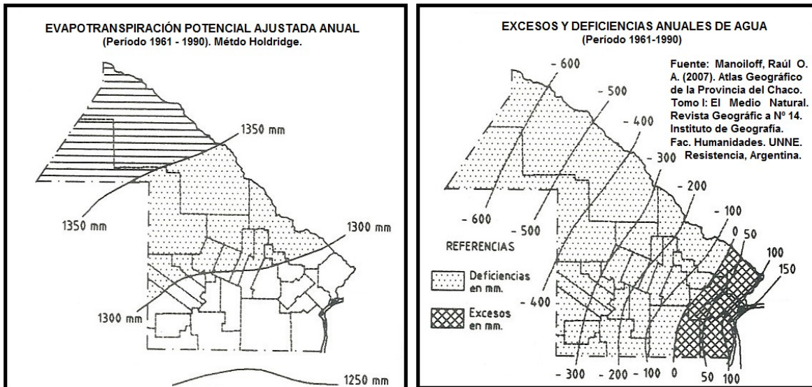
Mapas N° 4 y 5: Evapotranspiración potencial, excesos y deficiencias anuales de agua en el Chaco.
