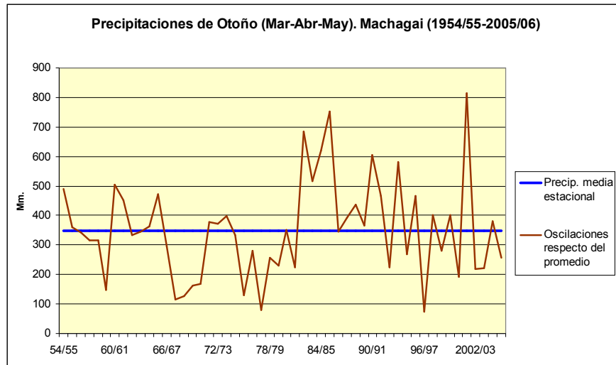
Gráfico N° 4: Precipitaciones en Otoño 1954-2006.
