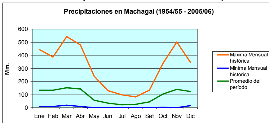
Gráfico N° 1: Precipitaciones mensuales máximas, medias y mínimas.
