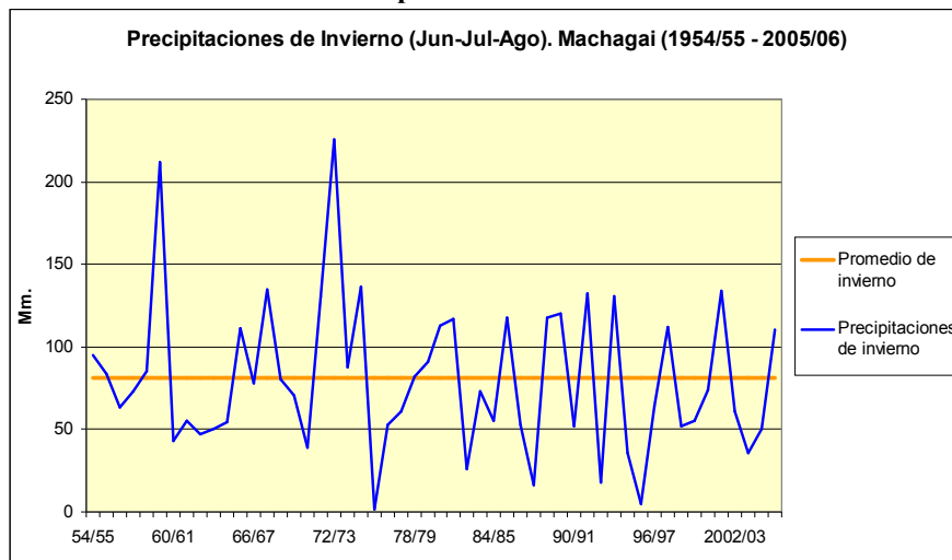
Gráfico N° 5: Precipitaciones en Invierno 1954-2006.
