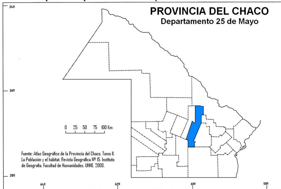
Mapa N° 1: Departamento 25 de Mayo en la Provincia del Chaco.
