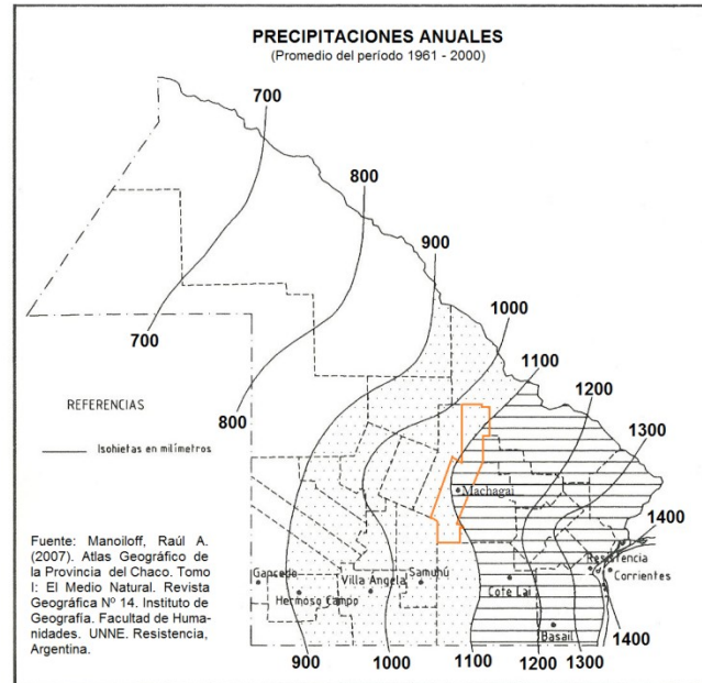
Mapa N° 3: Isohietas en la Provincia del Chaco.
