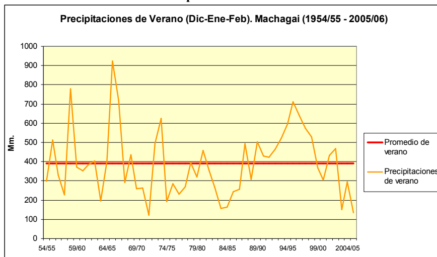
Gráfico N° 7: Precipitaciones en Verano 1954-2006.
