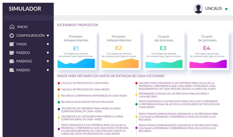
Fig. 9. Pantalla principal de la plataforma.
