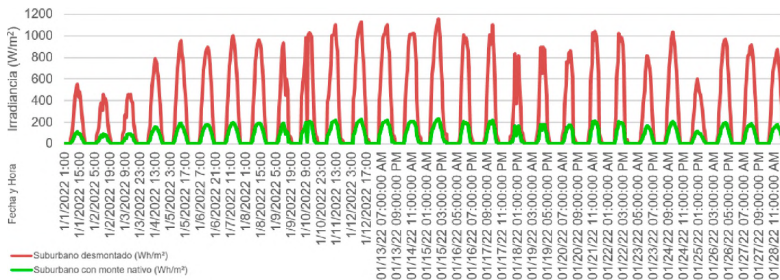
Figura 6: Irradiancia ( \text{Wh/m}^2 ) en el período monitoreado en el entorno descampado y corrección de valores para el entorno con monte nativo. Fuente: Elaboración autores.
