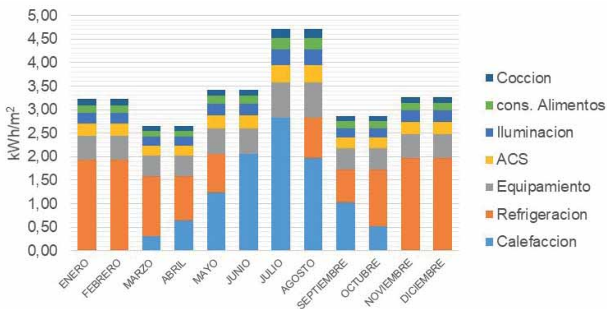
Gráfico 3. Curva de consumos del vector de energía eléctrica por mes, en el período 2015 a la actualidad. Fuente: elaboración propia
