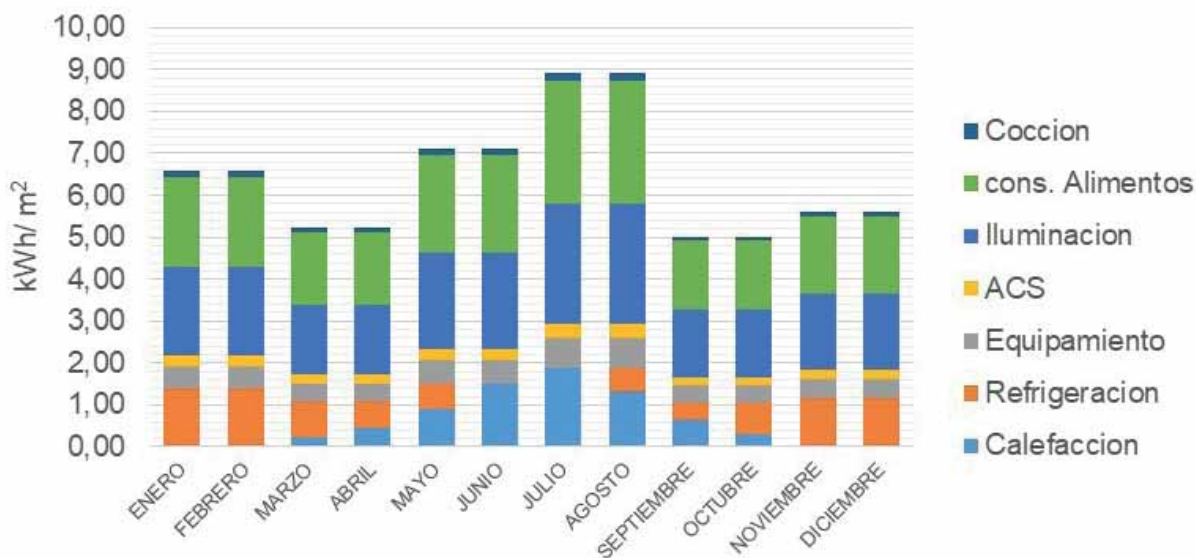
Gráfico 2. Curva de consumos del vector de energía eléctrica por mes, en el periodo 2005 a 2015. Fuente: elaboración propia
