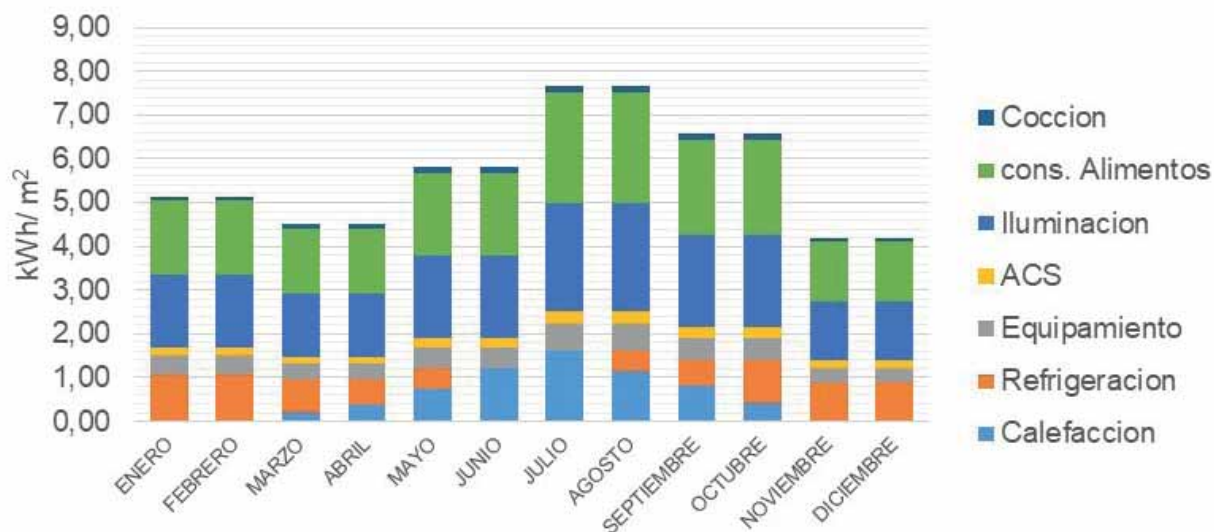
Gráfico 1. Curva de consumos del vector de energía eléctrica por mes, en el periodo 2002 a 2005. Fuente: elaboración propia
