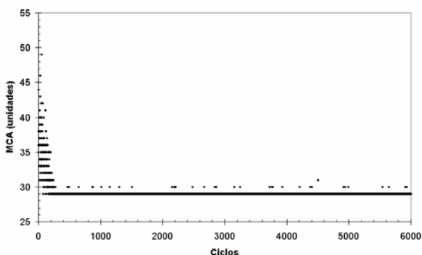
Fig. 7 - Custo acumulado do caminho de menor custo (MCA) em função do número de ciclos no problema 2.
