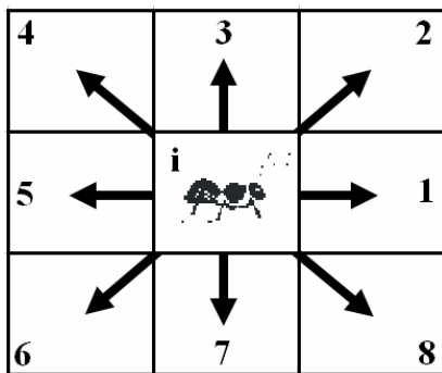
Fig. 2 - Janela de 3x3 celas para escolha da direção e sentido de avance de uma formiga artificial numa iteração.
