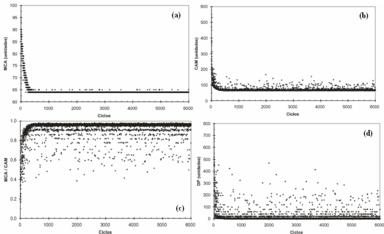
Fig. 5 - Resultados do primeiro problema em função do número de ciclos: (a) Custo acumulado do caminho de menor custo (MCA); (b) Custo acumulado médio dos caminhos definidos pela colônia de formigas (CAM); (c) Relação MCA/CAM; (d) Desvio padrão do custo acumulado dos caminhos da colônia de formigas (DP).
