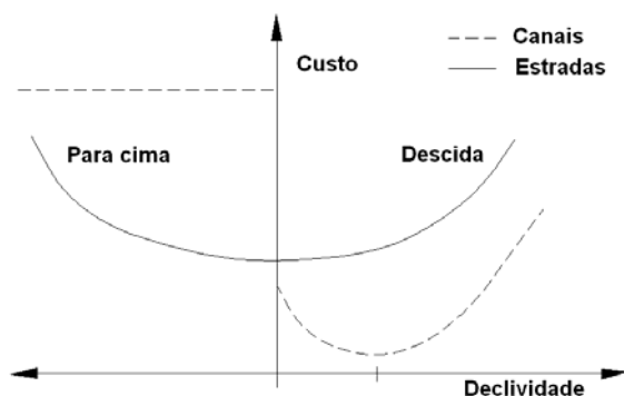
Fig. 12 - Forma geral da função custo incremental vs declividade para um canal de irrigação (linha tracejada) e para estradas (linha contínua).
