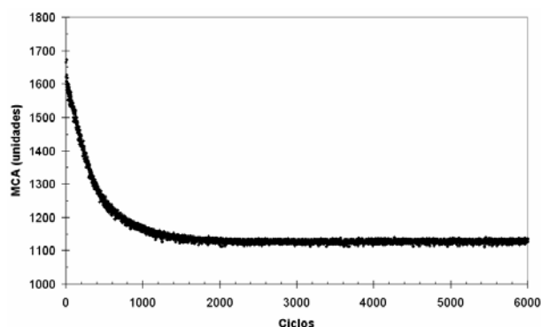
Fig. 9 - Custo acumulado do caminho de menor custo (MCA) em função do número de ciclos no problema do labirinto.
