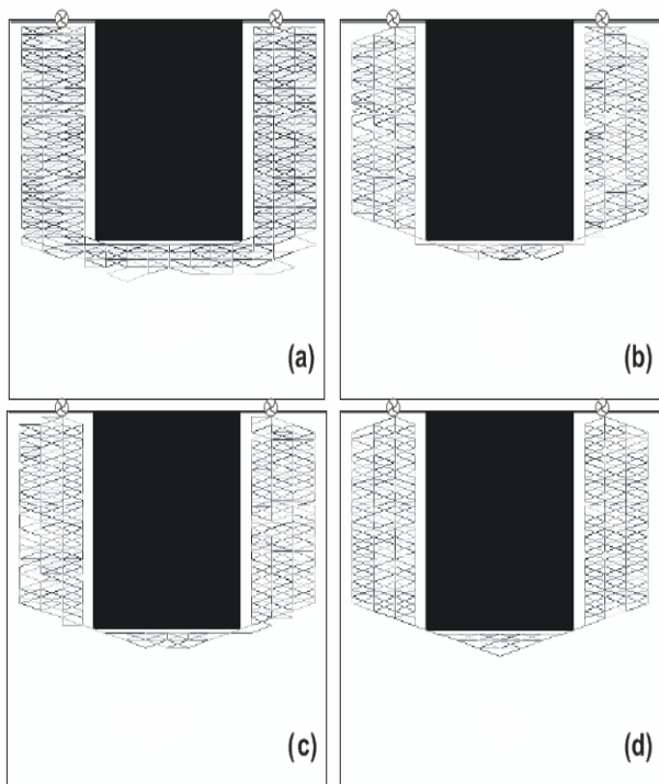
Fig. 4 – Caminhos de mínimo custo obtidos no primeiro problema em função do número de ciclos: (a) até o ciclo 500; (b) entre o ciclo 501 e 1000; (c) entre o ciclo 1001 e 2000; (d) resultados obtidos depois de 6000 ciclos.
