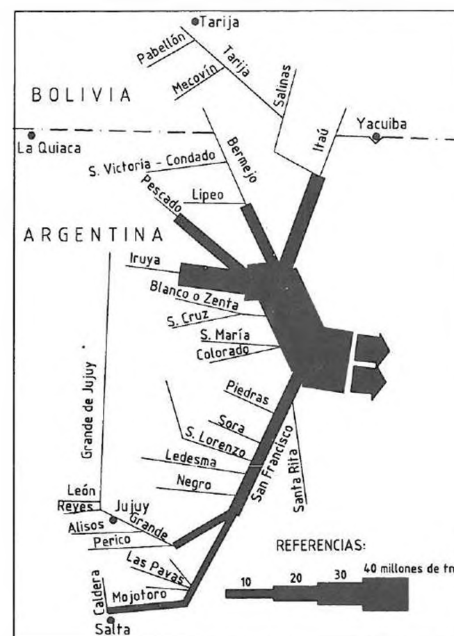
ESQUEMA DEL CAUDAL SÓLIDO ANUAL DEL RÍO BERMEJO Y DE SUS PRINCIPALES AFLUENTES
