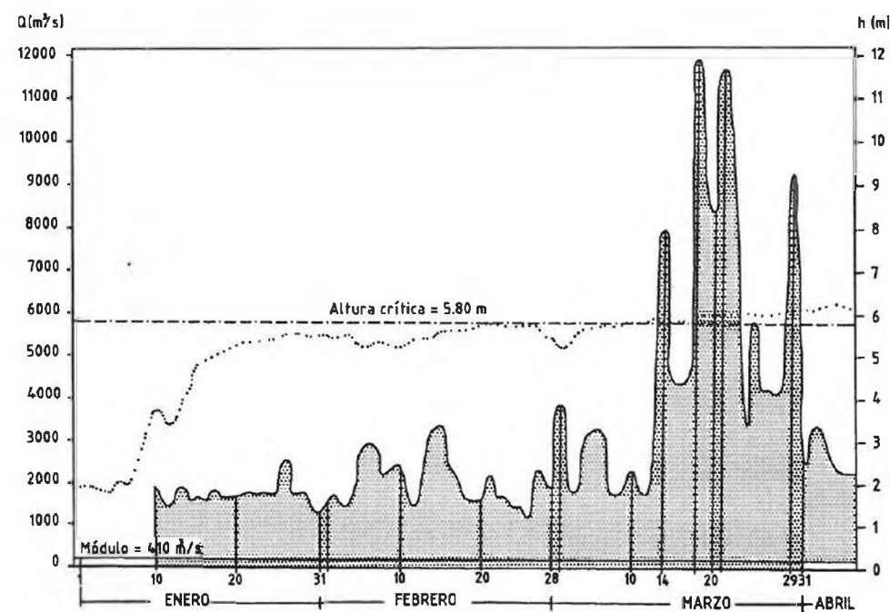
HIDROGRAMA DE LA CRECIDA DEL RÍO BERMEJO DURANTE EL PERÍODO 1983-1984
