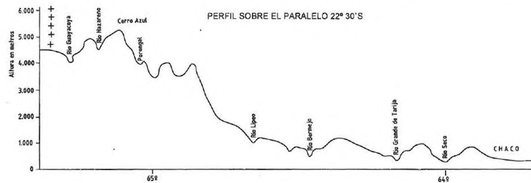
PERFILES TOPOGRÁFICOS DE LA ALTA CUENCA DEL BERMEJO
