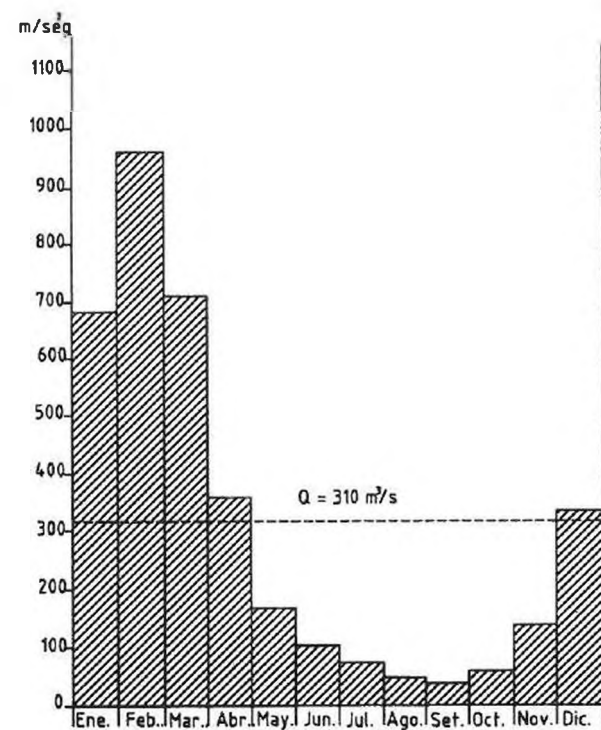
CAUDALES MEDIOS MENSUALES DEL RÍO BERMEJO EN ZANJA DEL TIGRE
