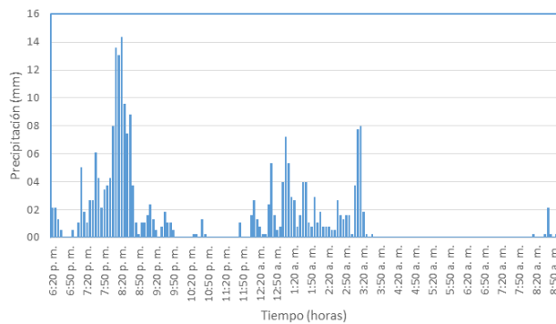
Figura 4. Hietograma de la tormenta registrada entre la noche del día 8 y la mañana del día 9 de enero de 2019 en el Campus Resistencia de la UNNE.
