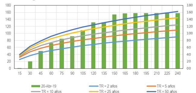
Figura 6. Láminas de precipitación (en mm) para diferentes TR comparadas con el hietograma del evento del sábado 20 de abril, según los registros de la Estación Zabala, en Avenida Ávalos, zona Carrefour.
