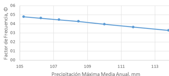
Figura 7. Tendencia del Factor de Frecuencia de Hershfield en función de la Precipitación Máxima Media Diaria para Resistencia, Estación Campus Resistencia-UNNE.
