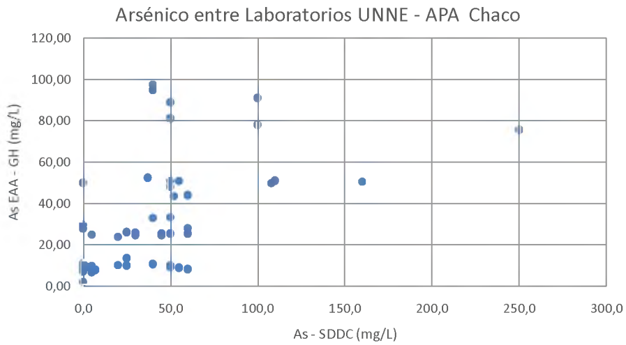
Figura 2. Gráfico de dispersión entre el laboratorio de Química de la UNNE y el laboratorio de APA-Chaco Fuente: Laboratorio de Química de la Facultad de Ingeniería de la UNNE y Laboratorio de APA-Chaco
