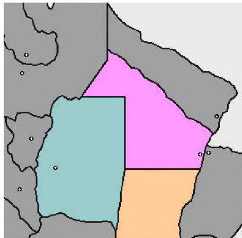
Figura 1. Ubicación de las provincias donde se realizaron los muestreos: Chaco y Santiago del Estero. Fuente: Academia de Ciencias Luventicus
