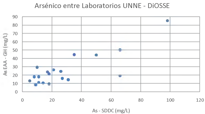
Figura 3. Gráfico de dispersión entre el Laboratorio de Química de la UNNE y el Laboratorio de DiOSSE-Santiago del Estero. Fuente: Laboratorio de Química de la Facultad de Ingeniería de la UNNE y Laboratorio de DiOSSE-Santiago del Estero
