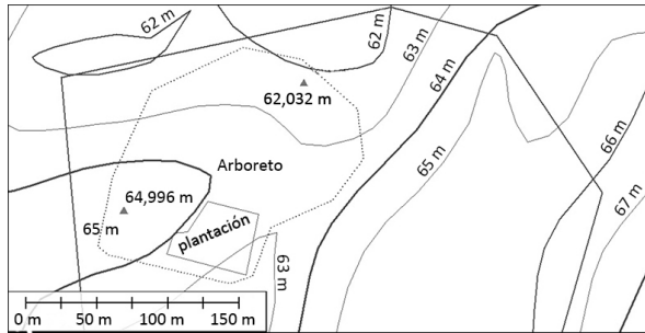
Figura 2. Curvas de nivel del área de interés a través de Global Mapper . Se señalan los puntos más alto y más bajo del terreno (Δ).
