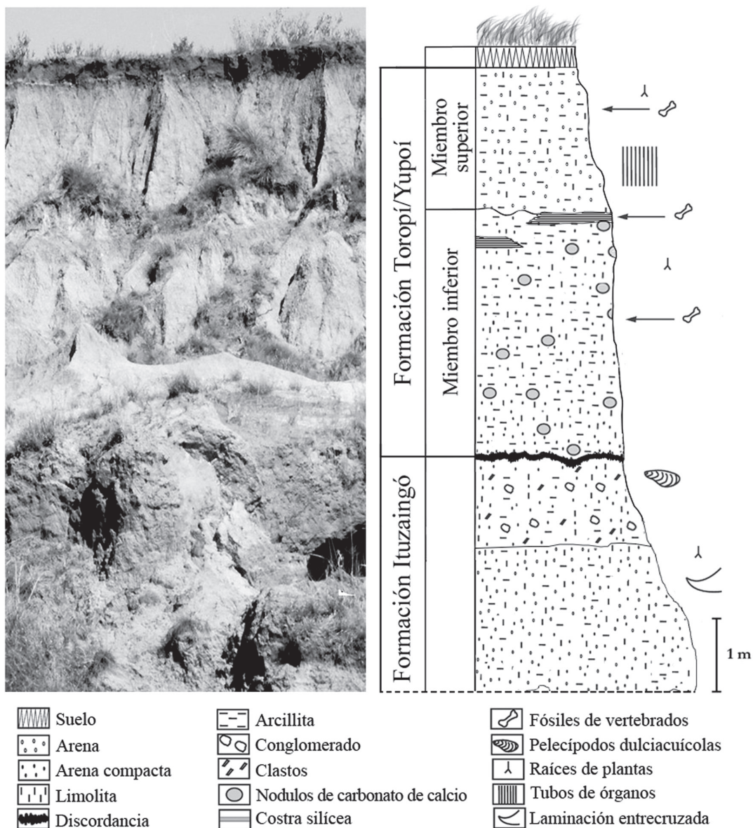
Figura 2. Perfil estratigráfico generalizado de la Formación Toropí/Yupoí y Formación Ituzaingó elaborado a partir de las descripciones litológicas de Herbst (1971) e Iriando (2010) (modificado de Zacarías et al. , 2013).
