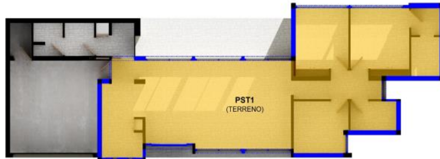
Figura 18: Identificación de los elementos de la envolvente térmica. Solado. Fuente: Anexo A, MAP(C) 2020
