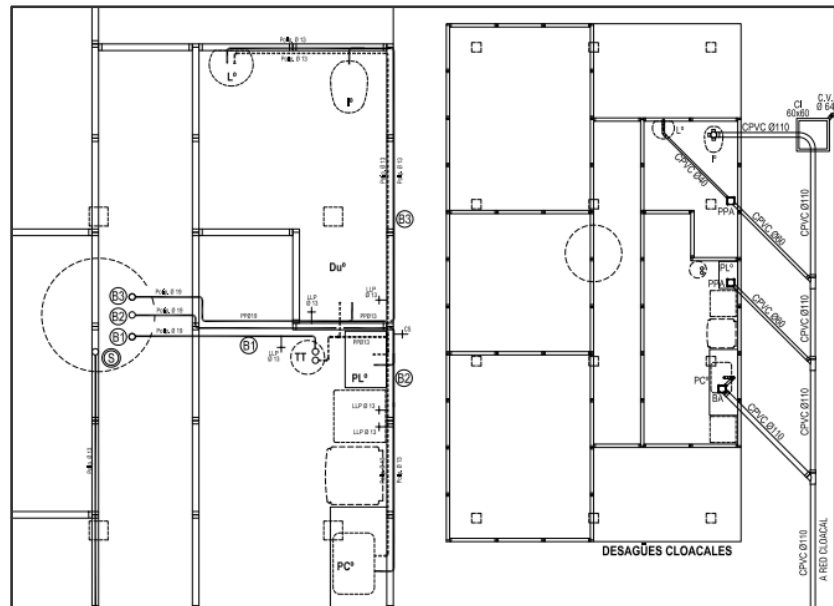
Figura 37: Instalación sanitaria: agua y cloacal. Fuente: Legajo técnico INVICO
