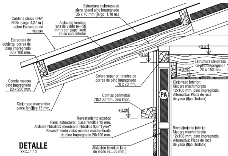
Figura 35: Detalle de encuentro de techo con muro y cielorraso.
