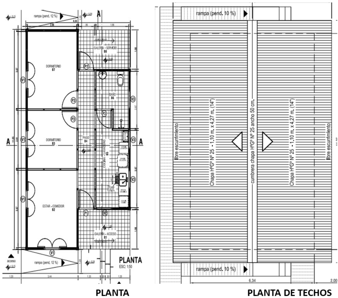
Figura 31: Planta principal de vivienda en madera. Fuente: Legajo técnico INVICO
