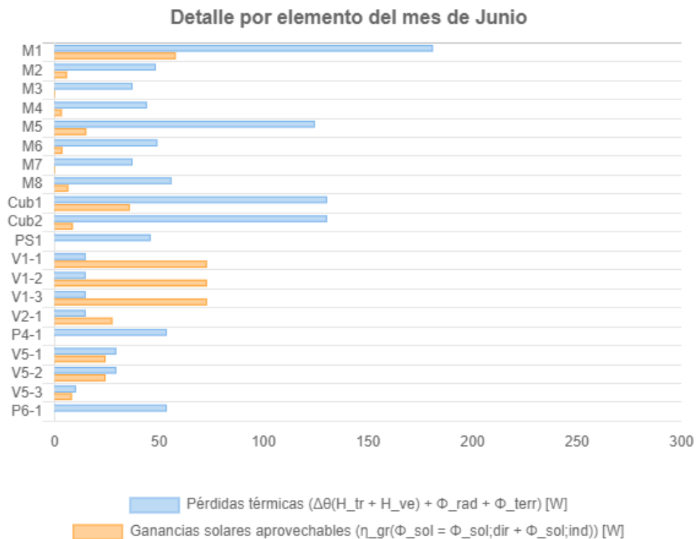
Figura 65: Pérdidas térmicas y ganancias solares aprovechables en mes de junio. Viv. de mampostería de ladrillos huecos. Fuente: Elaboración propia a través del Aplicativo informático para Etiquetado de Vivienda.
