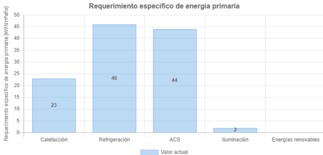
Figura 61: Requerimiento específico de energía primaria de vivienda de mampostería de ladrillos huecos. Calefacción, refrigeración, agua caliente sanitaria (ACS). Fuente: Elaboración propia a través del Aplicativo informático para Etiquetado de Vivienda.
