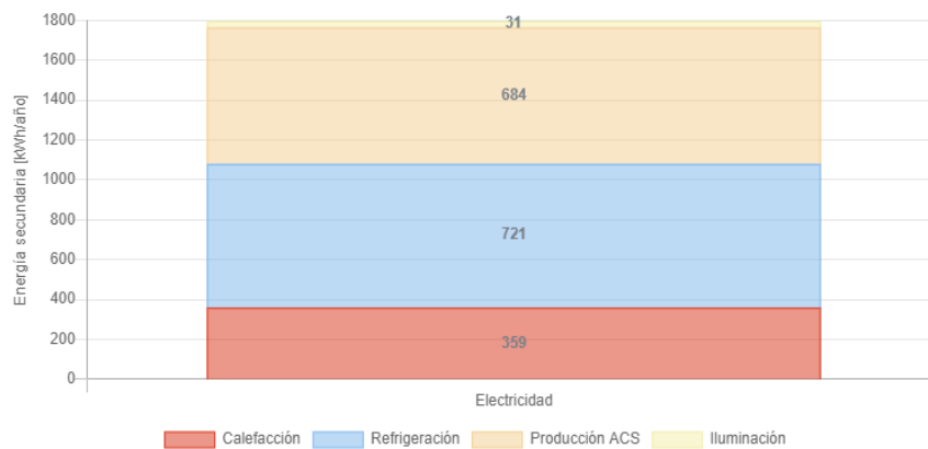
Figura 62: Requerimiento específico de energía secundaria de vivienda en mampostería de ladrillos huecos. Calefacción, refrigeración, ACS, iluminación. Fuente: Elaboración propia a través del Aplicativo informático para Etiquetado de Vivienda.
