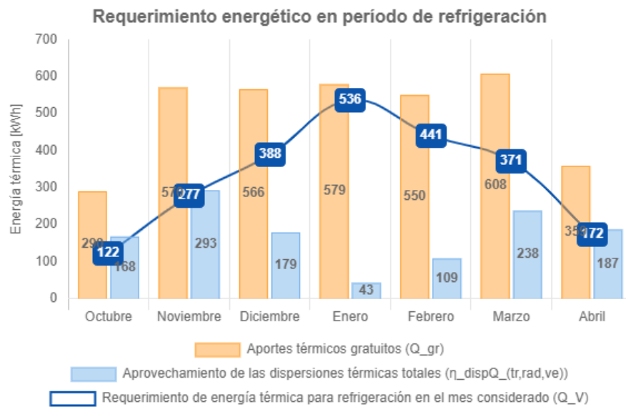
Figura 64: Requerimiento energético en periodo de refrigeración. Vivienda de mampostería de ladrillos huecos. Fuente: Elaboración propia a través del Aplicativo informático para Etiquetado de Vivienda.
