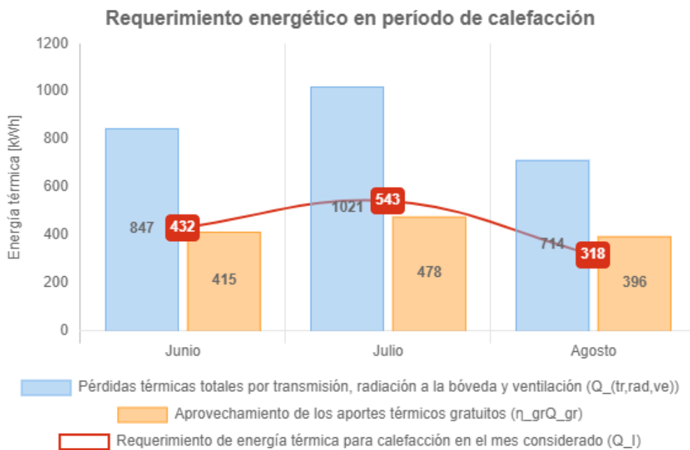
Figura 63: Requerimiento energético en período de calefacción. Vivienda de mampostería de ladrillos huecos. Fuente: Elaboración propia a través del Aplicativo informático para Etiquetado de Vivienda.
