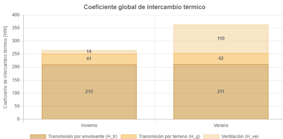
Figura 60: Coeficiente global de intercambio térmico de vivienda en mampostería de ladrillos huecos. Transmisión por envolvente terreno y ventilación. Fuente: Elaboración propia a través del Aplicativo informático para Etiquetado de Vivienda.
