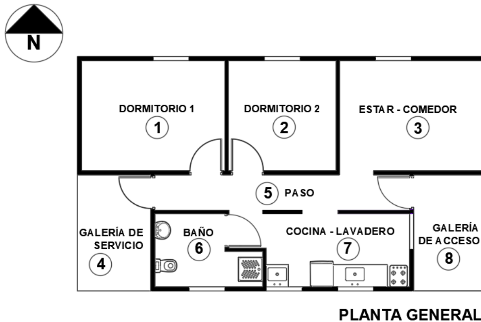
Figura 33: Planta principal de vivienda en madera. Fuente: Elaboración propia, datos Legajo técnico INVICO.
