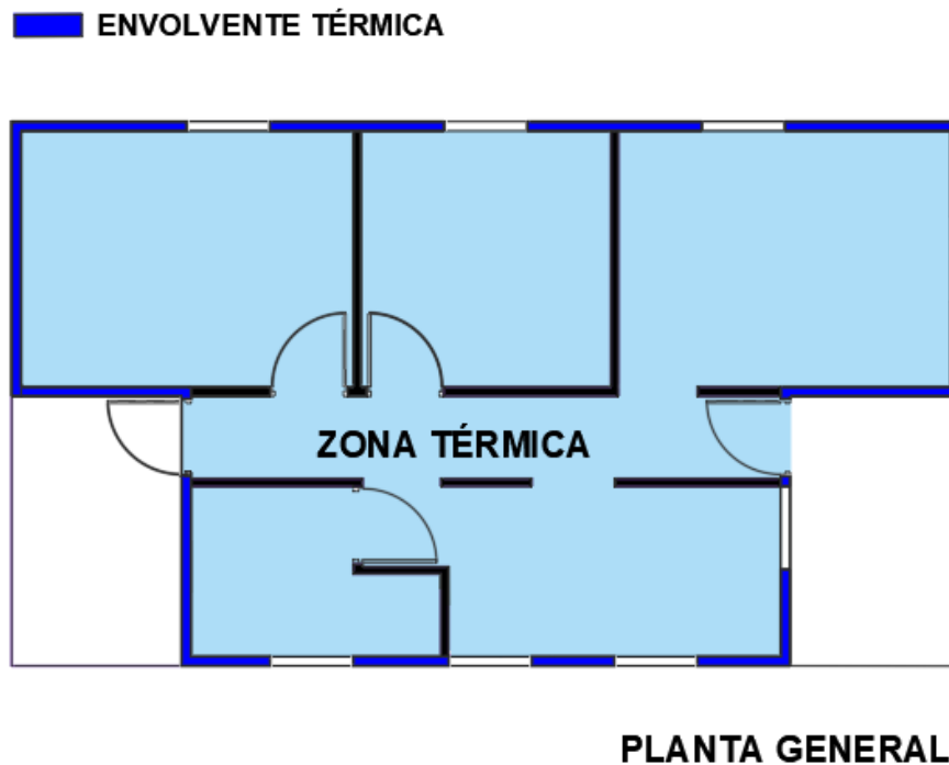
Figura 43: Cuarto paso: reconocimiento de la envolvente térmica. Fuente: Elaboración propia.
