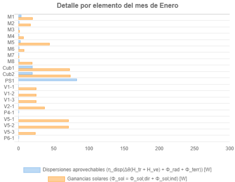
Figura 66: Dispersiones aprovechables y ganancias solares en mes de enero. Vivienda de mampostería de ladrillos huecos. Fuente: Elaboración propia a través del Aplicativo informático para Etiquetado de Vivienda.
