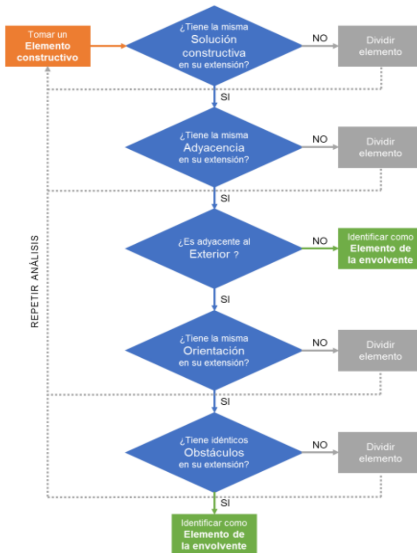
Figura 20: Diagrama de flujo para identificación de los elementos de la envolvente térmica. Fuente: Anexo A, MAP(C) 2020
