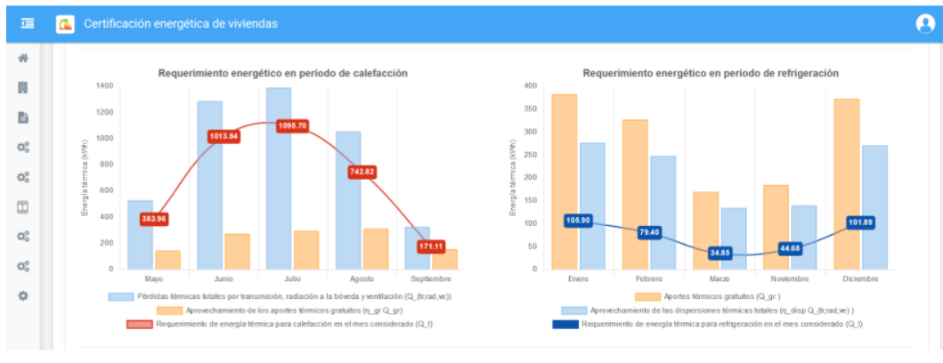
Figura 27: Datos de requerimientos energéticos en periodos de calefacción y refrigeración que arroja el sistema informático de etiquetado. Fuente: MAP(C) 2020.
