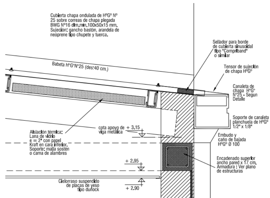
Figura 39: Detalle de encuentro de techo muro cielorraso. PT60. Fuente: Legajo técnico INVICO
