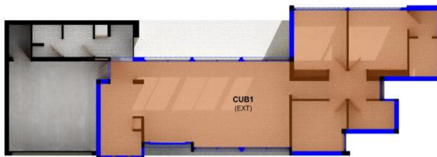
Figura 19: Identificación de los elementos de la envolvente térmica. Cubierta. Fuente: Anexo A, MAP(C) 2020
