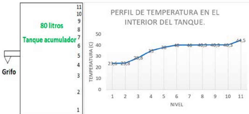
Figura 3: Medición de temperatura en el interior del tanque acumulador.
